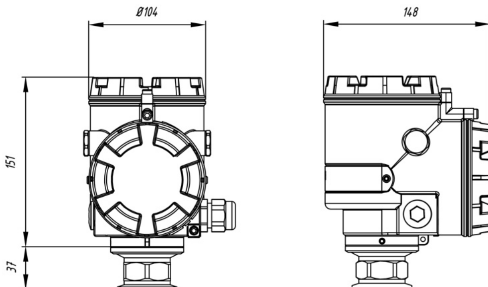
Рисунок Б.1.4.1 - Корпус уровнемера АльфаФлекс-Н52 из алюминиевого сплава с 2 отсеками с исполнением «Л: Viton; -40...+80 гpC», «М: Viton; -40...+150 гpC», «К: Kalrez; -20...+200 гpC»
