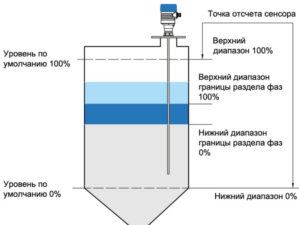
Рисунок 17 – Диапазон измерения
